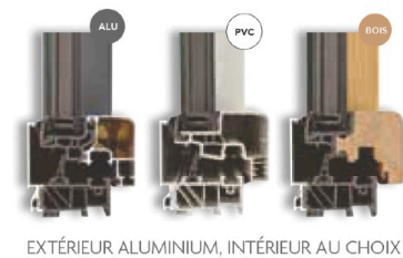
EXTÉRIEUR ALUMINIUM, INTÉRIEUR AU CHOIX
