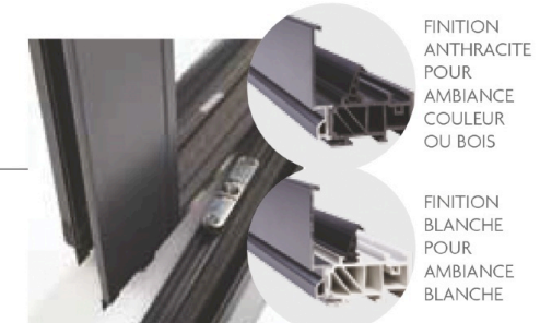
POSE AVEC JOINT THERMO-ACOUSTIQUE EN OPTION (PERMET DE MASQUER LES VIS DE FIXATION) POSE SANS JOINT THERMO-ACOUSTIQUE
